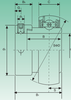
SA 2 anello esterno sferico outer spherical ring
