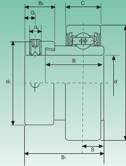
SA 2C anello esterno cilindrico outer cylindrical ring
